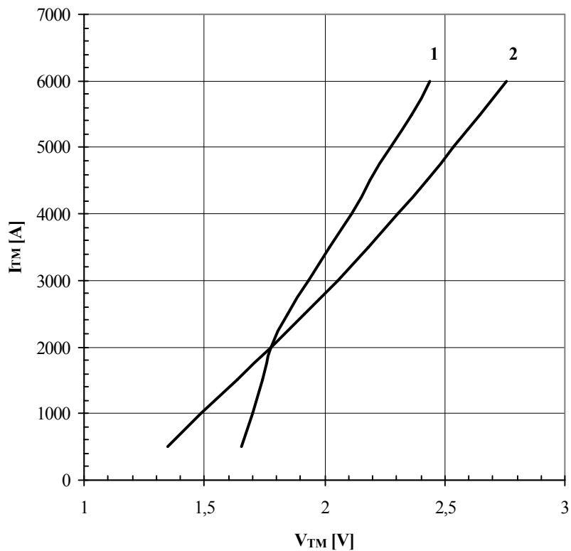
Рис.1 – Предельная вольт-амперная характеристика. 1 – T j =25 °C 2 – T j =125 °C
