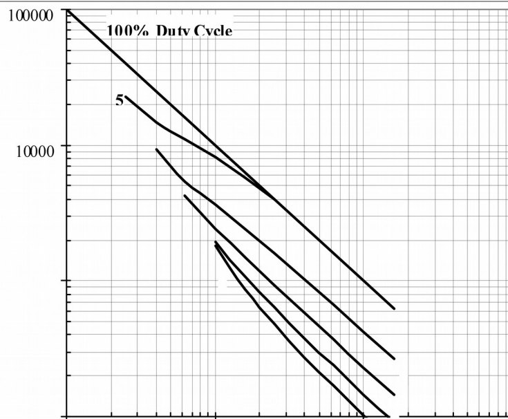
Рис. 14 — Зависимость частоты прямоугольных импульсов тока от длительности импульсов
