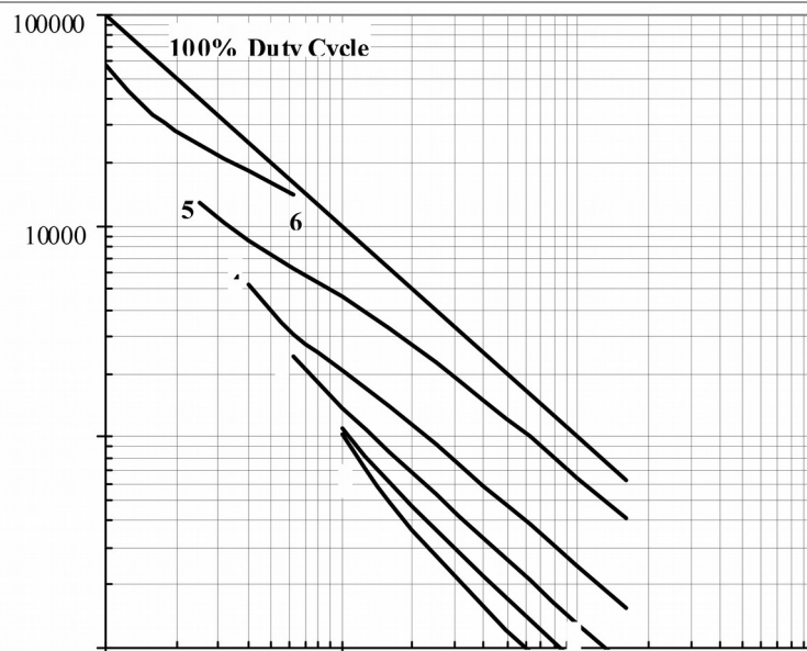
Рис. 16 — Зависимость частоты прямоугольных импульсов тока от длительности импульсов
