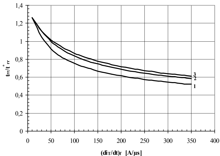
Рис. 8 — Зависимость времени обратного восстановления t_{rr} от скорости спада анодного тока di_T/dt
