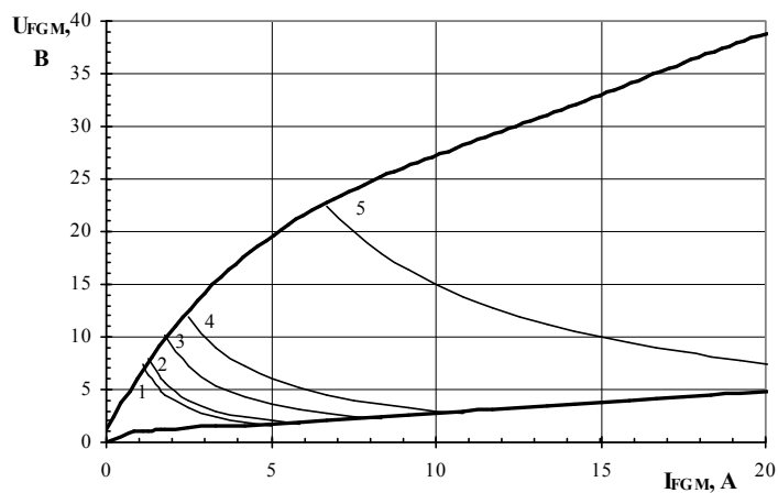
Максимальные потери мощности цепи управления
