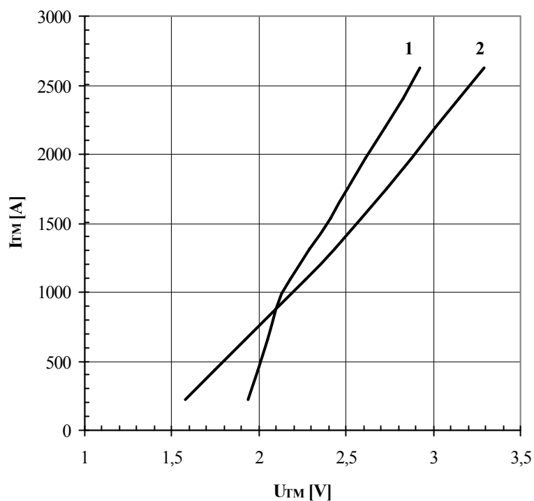
Рис.1 – Предельная вольт-амперная характеристика. 1 – T_j=25\text{ }^\circ\text{C} 2 – T_j=125\text{ }^\circ\text{C}
