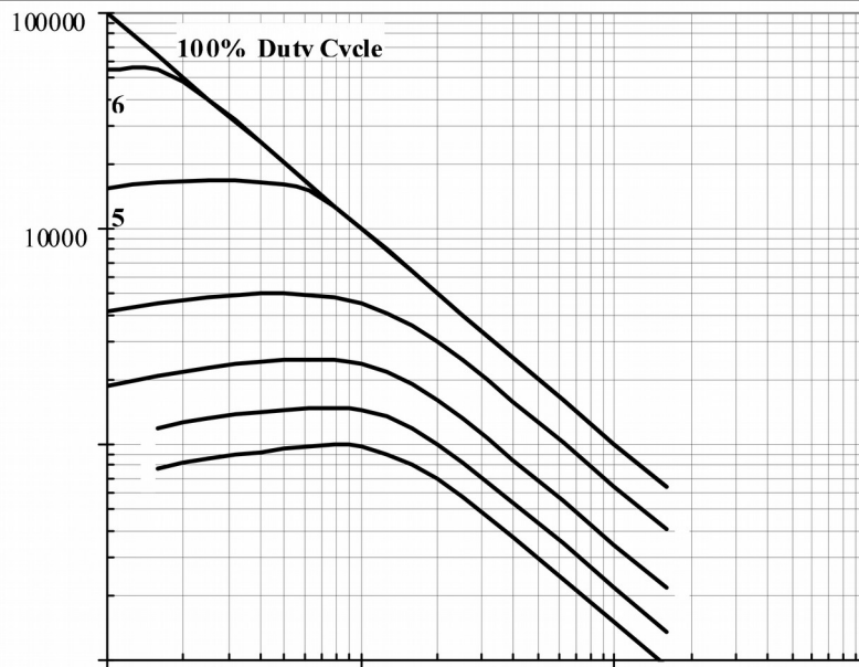
Рис. 10 — Зависимость частоты синусоидальных импульсов тока от длительности импульсов тока
