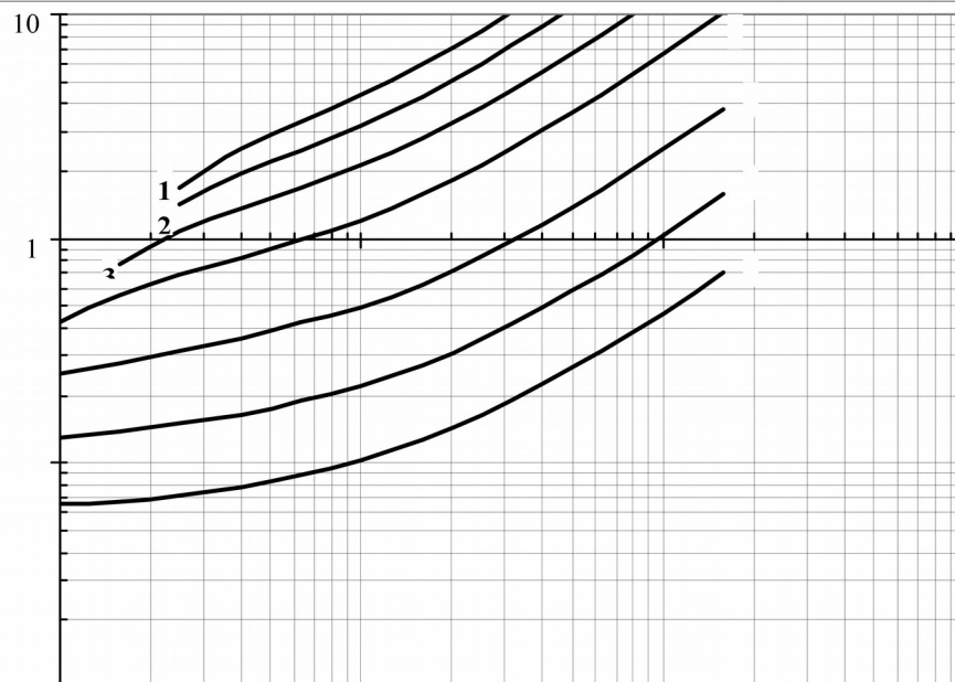
Рис. 27 – Зависимость энергии потерь за один синусоидальный импульс тока от длительности импульса
