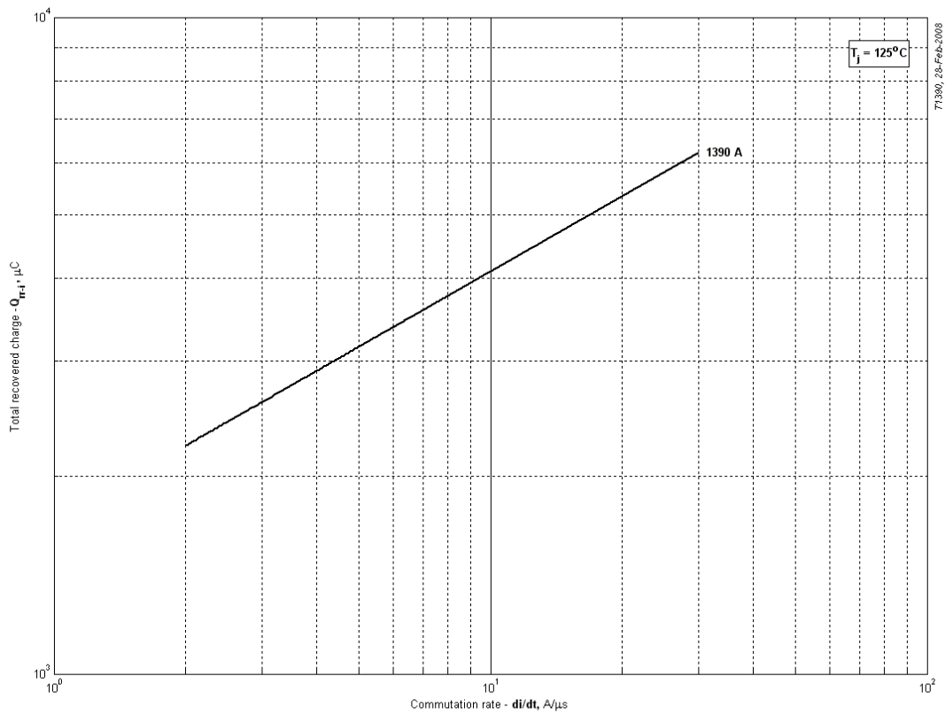
Рис. 5 - Заряд обратного восстановления, Q_{rr-i}
