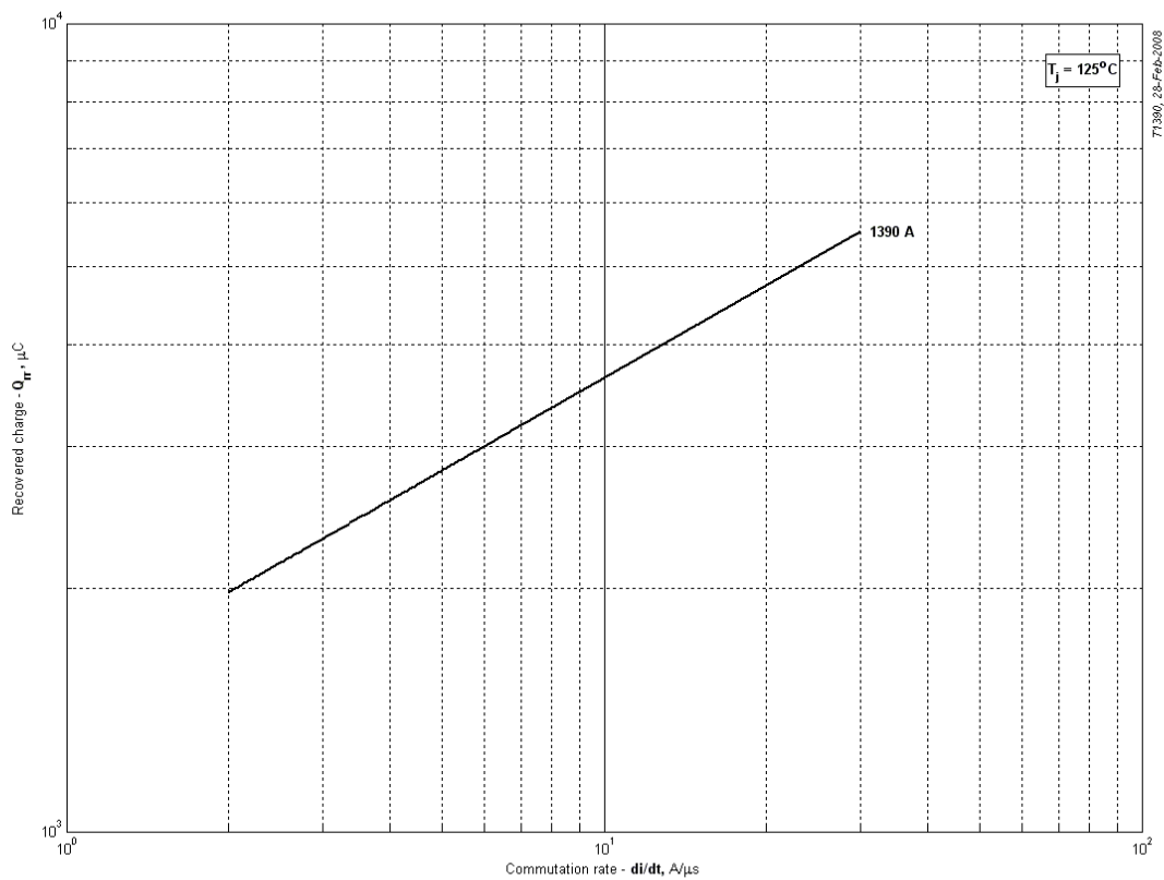
Рис. 6 - Заряд обратного восстановления, Q_{rr} (линеризованный)
