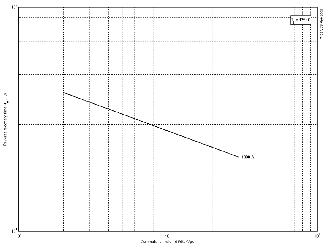
Рис. 8 - Максимальное время обратного восстановления, t_{tr} (линеризованный)
