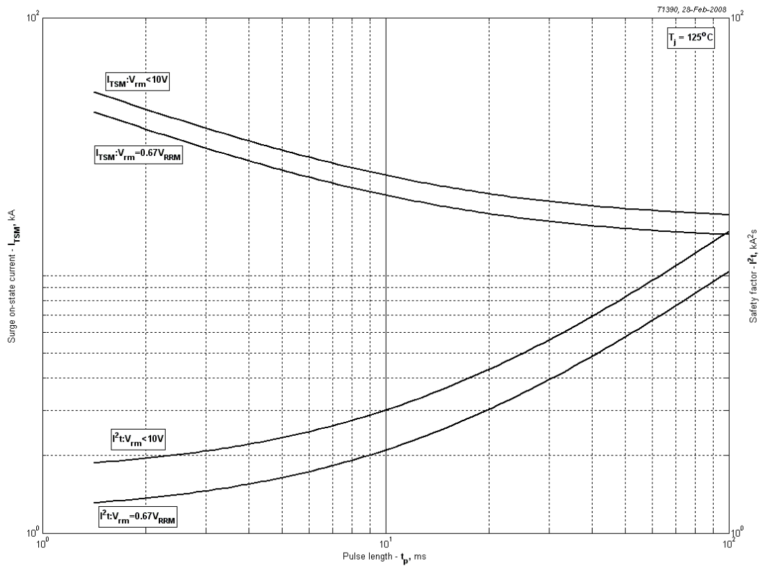
Рис. 13 – Максимальные ударные и I^2t характеристики
