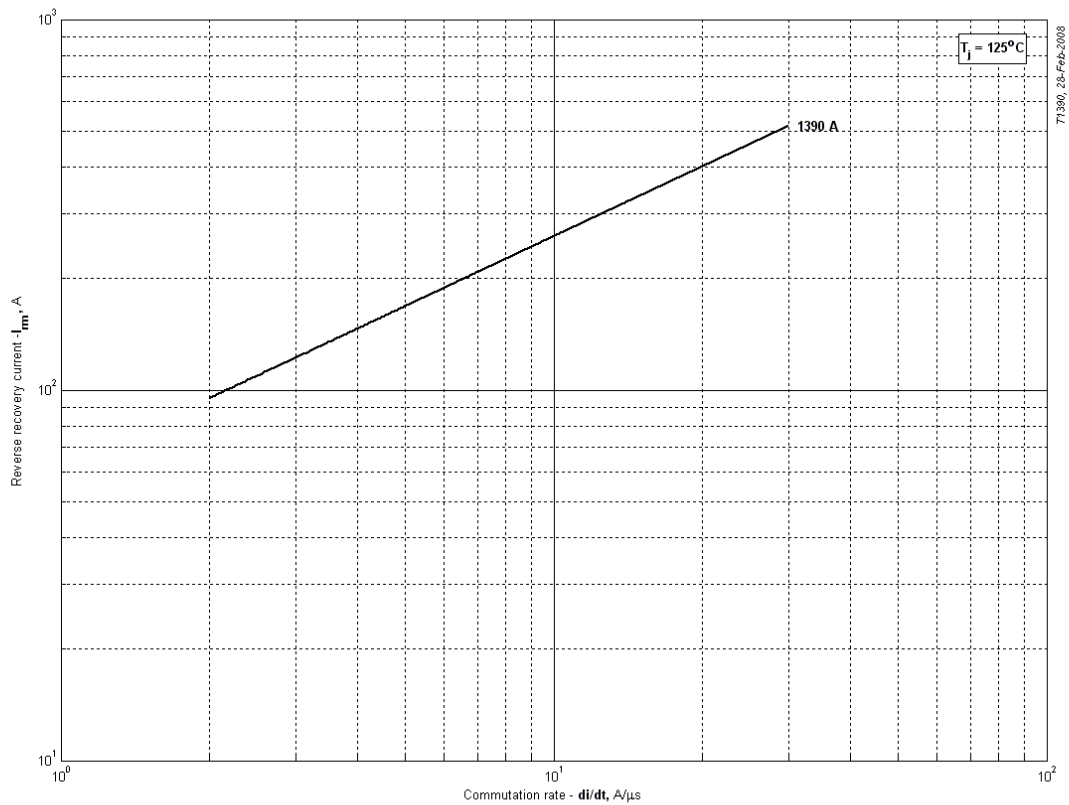
Рис. 7 - Максимальный обратный ток восстановления, I_{rm}
