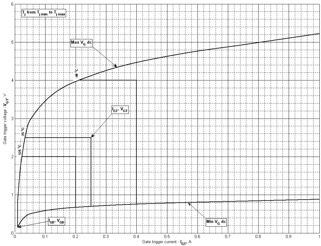
Рис. 3 – Вольт – амперная характеристика цепи управления – границы переключения
