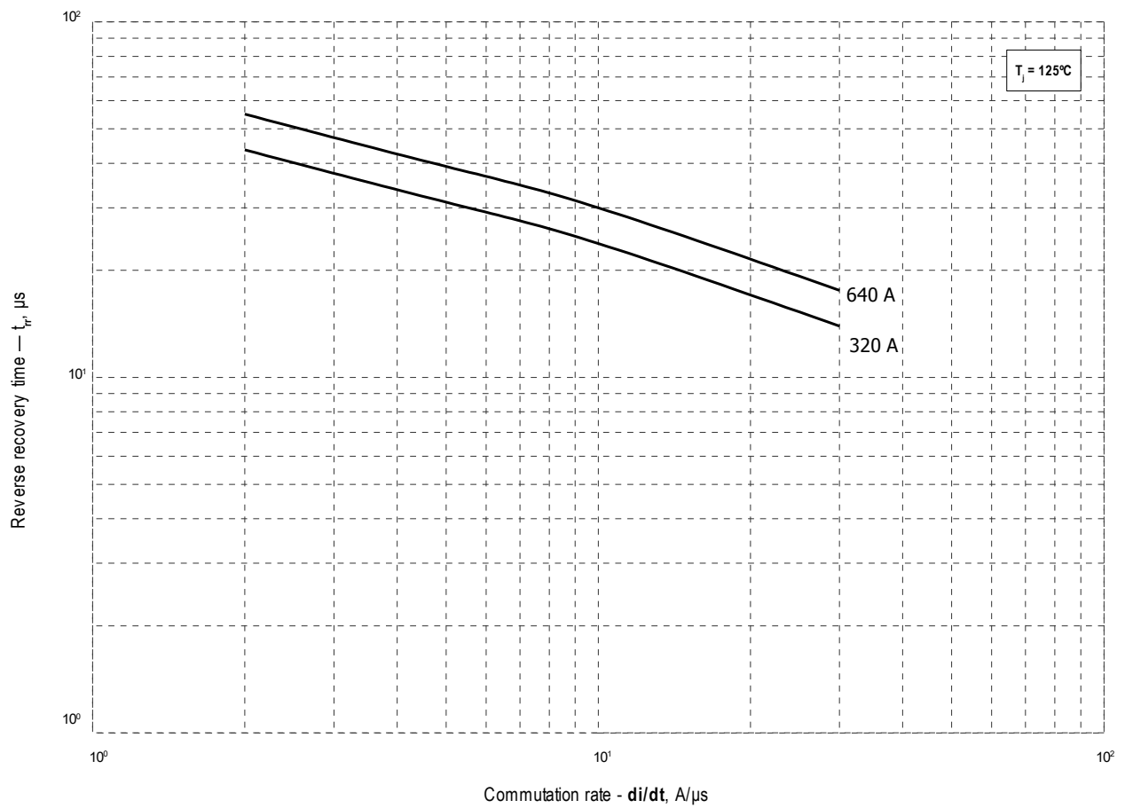
Рис. 8 – Максимальное время обратного восстановления, t_{rr} (по ГОСТ 24461, хорда 25%)
