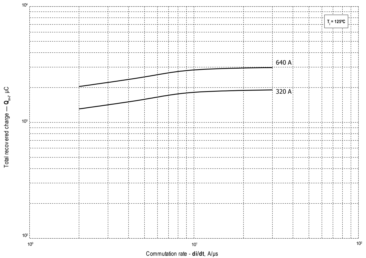
Рис. 5 – Максимальный интегральный заряд обратного восстановления, Q_{rr-i}
