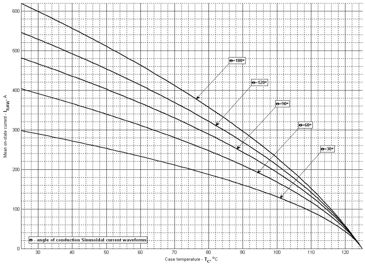
Рис. 11 - Зависимость среднего прямого тока I_{FAV} от температуры корпуса T_C для синусоидальной формы тока при различных углах проводимости ( f=50 Гц)
