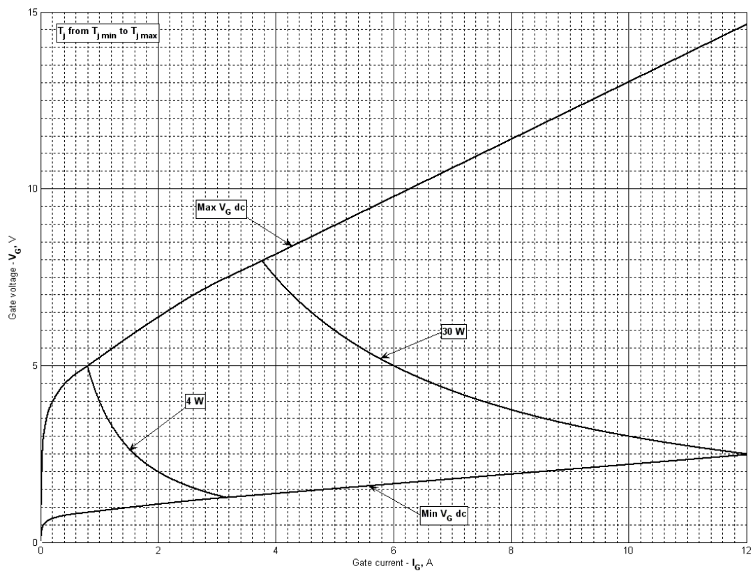
Рис. 4 – Вольт – амперная характеристика цепи управления
