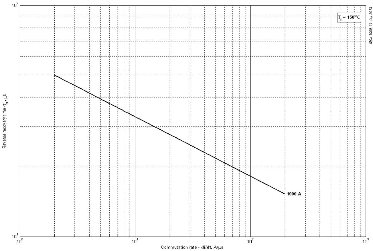
Рис. 6 – Максимальное время обратного восстановления, t_{tr} (по ГОСТ 24461, хорда 25%)
