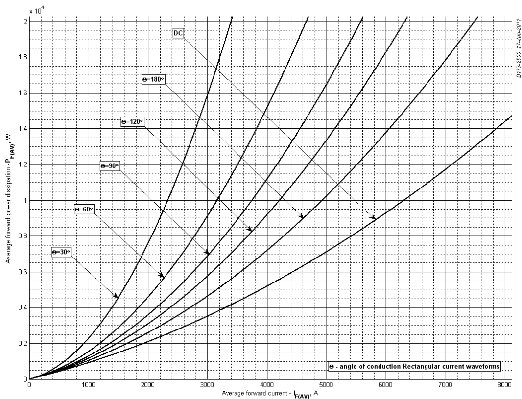
Рис. 8 – Зависимость потерь мощности P_{FAV} от среднего прямого тока I_{FAV} прямоугольной формы при различных углах проводимости ( f=50 Гц, двустороннее охлаждение)
