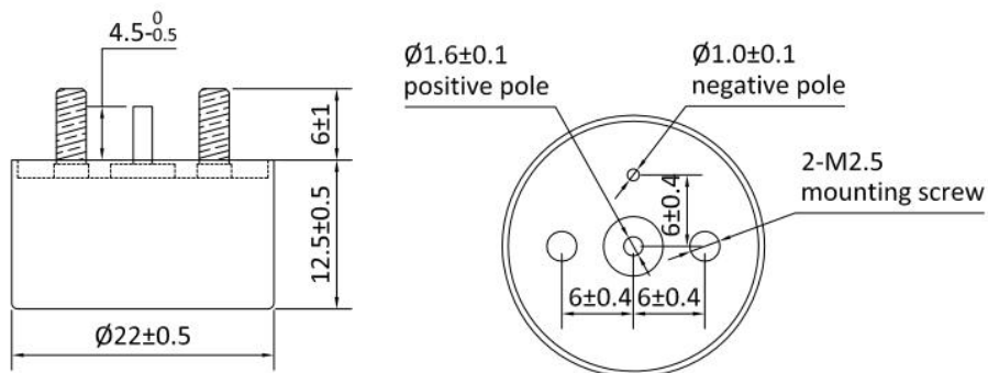
THC1W Ø22X12.5 Layout
